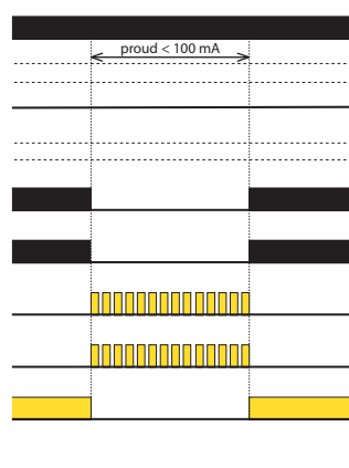
pokles (výpadek) proudu
